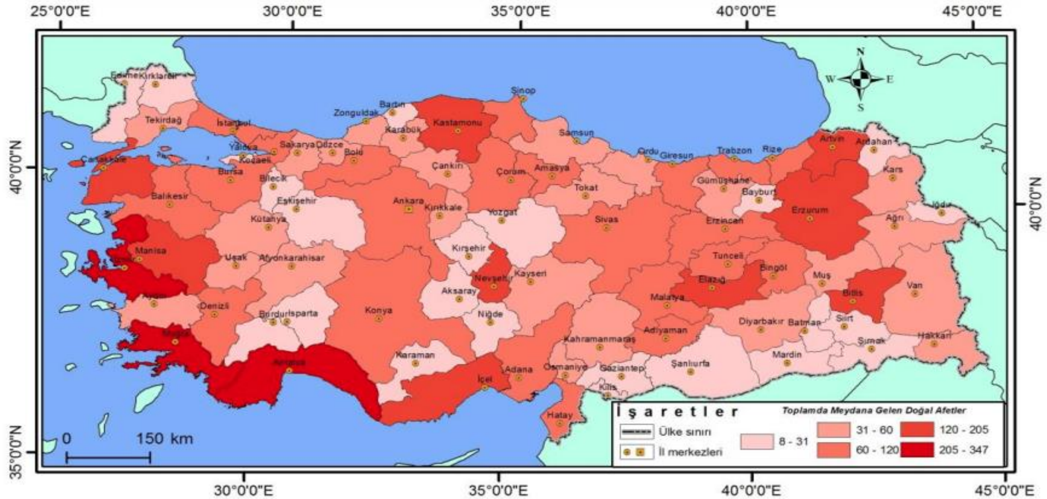
Şekil 1. Türkiye'nin konumu ve toplamda yaşanmış doğal afetlerin dağılışı (1970-2012)
